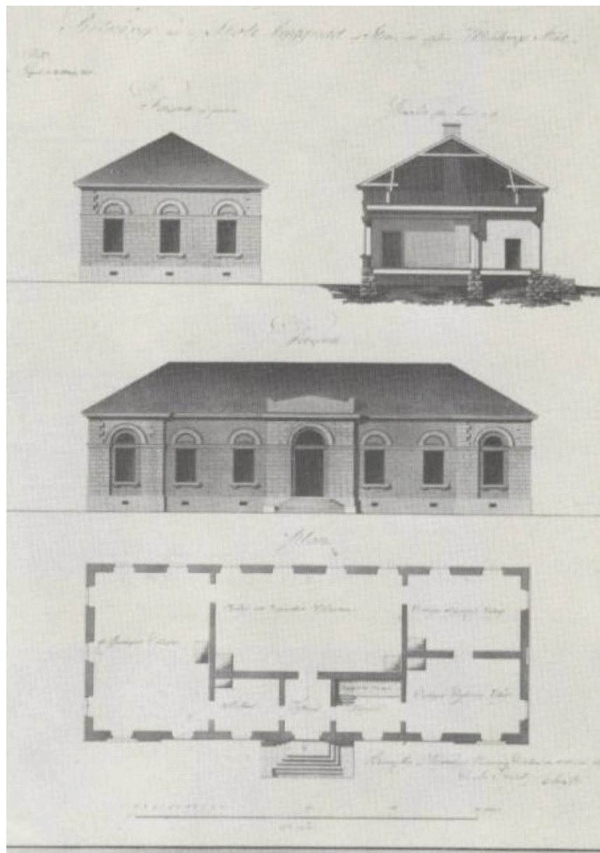
Kuva 40. Oulun triviaalikoulu. Intendentinkonttorin suunnitelma virakennusta varten vuodelta 1825. Konseptipiirustus. Raki
